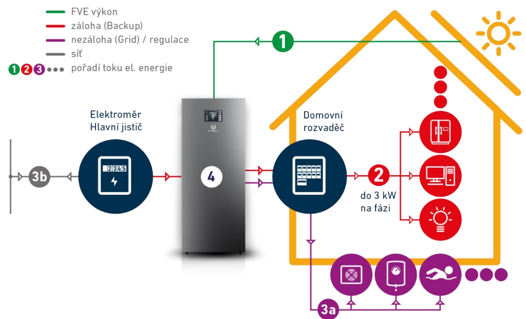
Obr. 21 – Znárodnění toku energie v objektu v režimu HOME GRID IV - UPS
