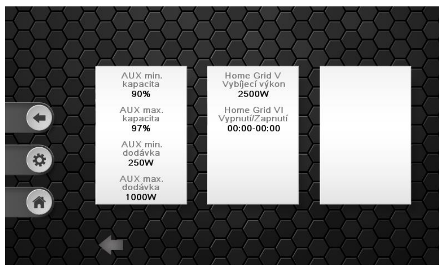
Obr. 28 – okno expertní nastavení pro AUX
