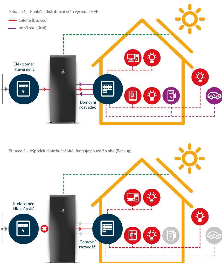
Obr. 5 – Schéma zapojení okruhů Záloha a Nezáloha při dostupné distribuční síti
