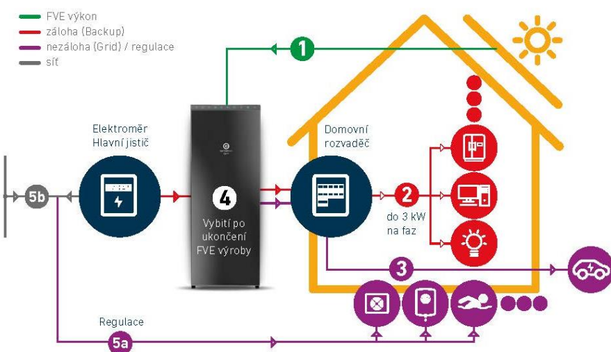
Obr. 13 – Znázornění toku energie v objektu v režimu HOME GRID II.
