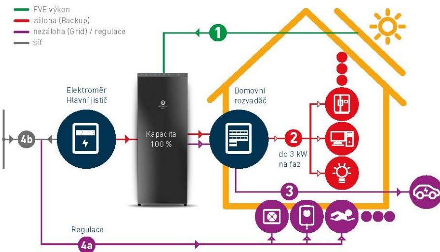
Obr. 15 – Znáznornění toku energie v objektu v režimu HOME GRID IV - UPS
