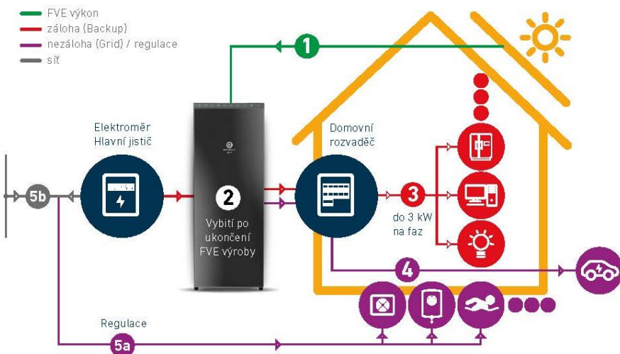
Obr. 14 – Znáznornění toku energie v objektu v režimu HOME GRID III.
