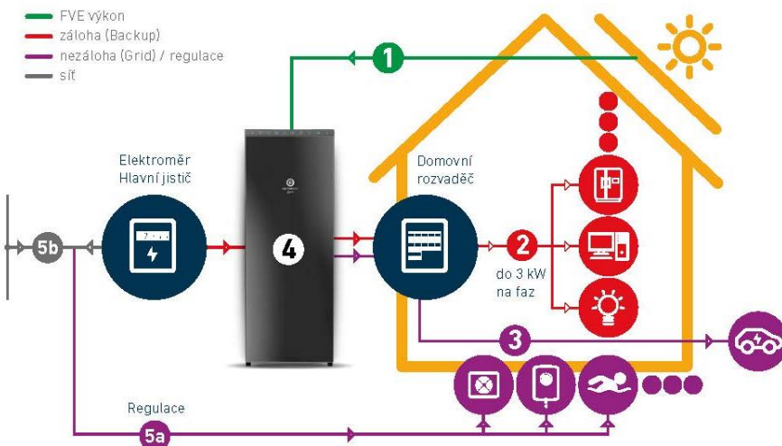
Obr. 12 – Znázornění toku energie v objektu v režimu HOME GRID I.
