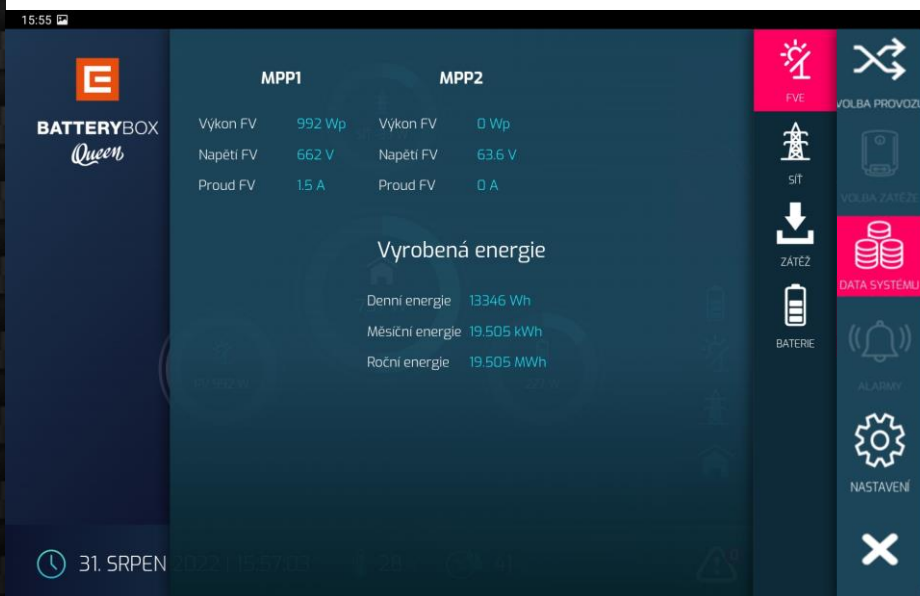
Obr. 17 – ukázka stavů v oddíle PV (Fotovoltaické panely) aplikace ČEZ BATTERY BOX Queen
