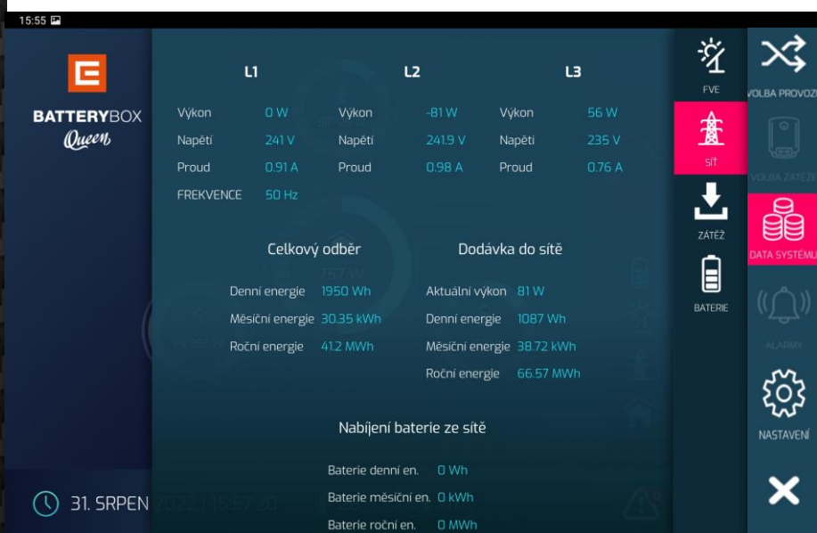
Obr. 18 – ukázka stavů v oddíle Sít aplikace ČEZ BATTERY BOX Queen
