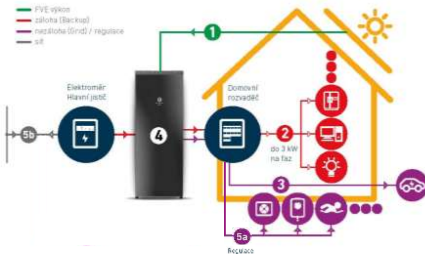
Obr. 14 – Znárodnění toku energie v objektu v režimu HOME GRID I. Pro soustavu TN-S
