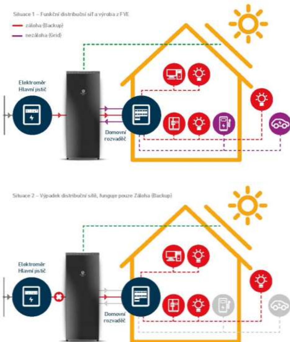
Obr. 6 – Schéma zapojení okruhů Záloha a Nezáloha při dostupné distribuční síti
