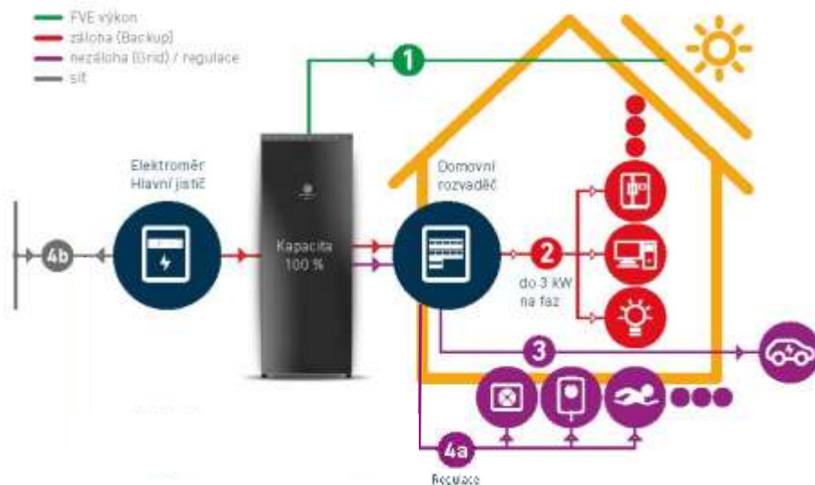
Obr. 16 – Znárodnění toku energie v objektu v režimu HOME GRID IV - UPS
