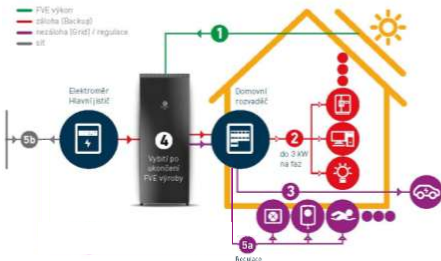
Obr. 15– Znáznornění toku energie v objektu v režimu HOME GRID II.
