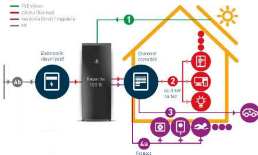
Obr. 16 – Znáznornění toku energie v objektu v režimu HOME GRID IV - UPS
